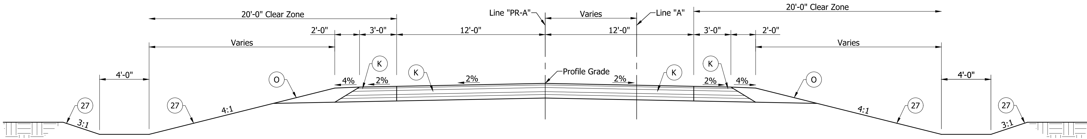
TYPICAL CROSS SECTION Scale: 1/4" = 1'-0" Sta. 14+07.00 "PR-A" to Sta. 95+20.08 "A"
