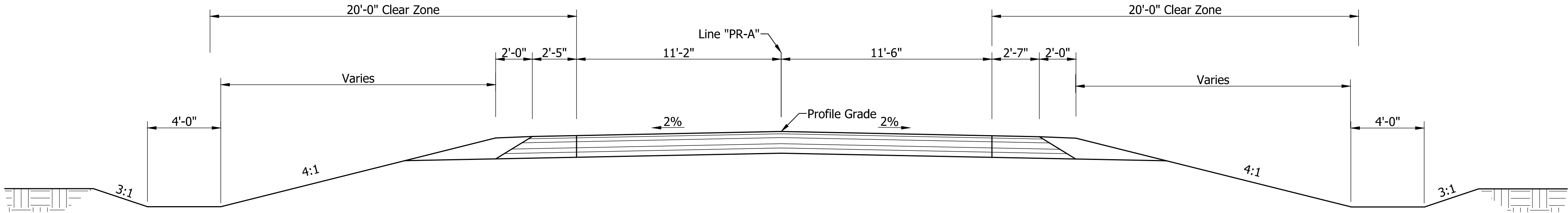
INCIDENTAL CONSTRUCTION TYPICAL CROSS SECTION Scale: 1/4" = 1'-0" Sta. 13+07.00 "A" to Sta. 14+07.00 "PR-A" Sta. 95+20.08 "A" to Sta. 95+70.00 "A"
